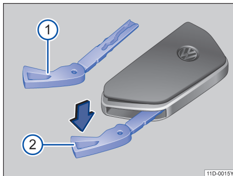
图 49 汽车钥匙：打开电池盒盖板
