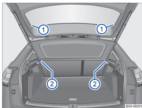
图 189 拆卸和安装行李厢盖板
