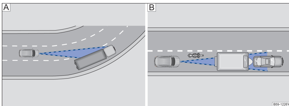
图 144 [A]. 处在弯道里的汽车；[B]. 前方行驶的摩托车处在雷达传感器探测范围外
