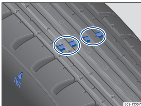
图 224 轮胎花纹磨损标记
