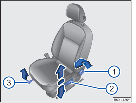
图 76 左侧前座椅上的操作元件
