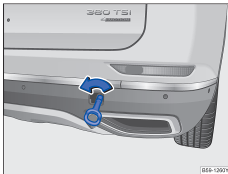
图 215 在保险杠右后部：安装牵引环
