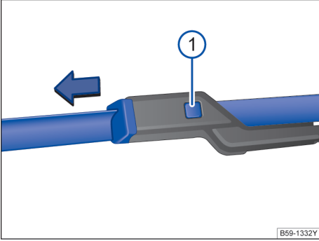
图 204 更换前风窗刮水器刮水片
