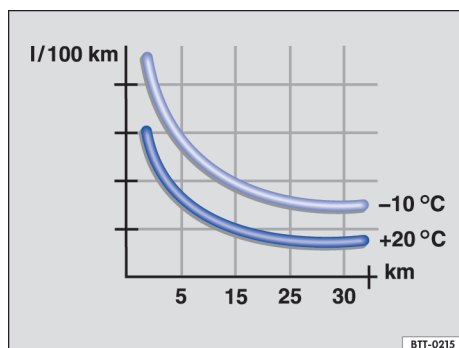
图 128 两种不同环境温度时的百公里油耗
