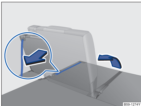
图 87 将第三排座椅翻回
