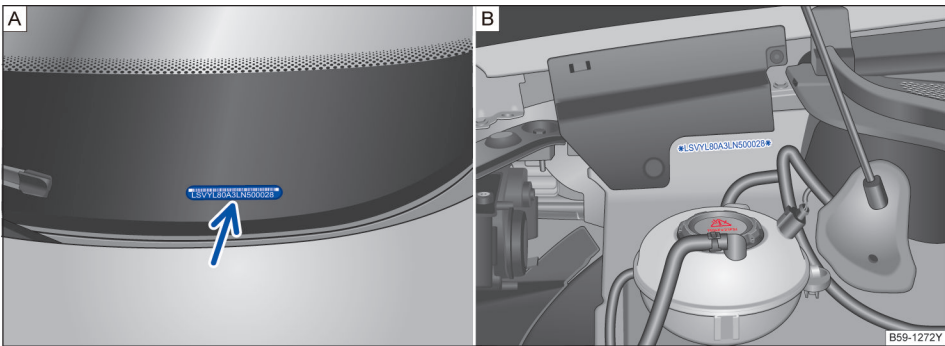
图 237 A. 车辆识别代号 B. 发动机舱内的车辆识别代号钢印位置
