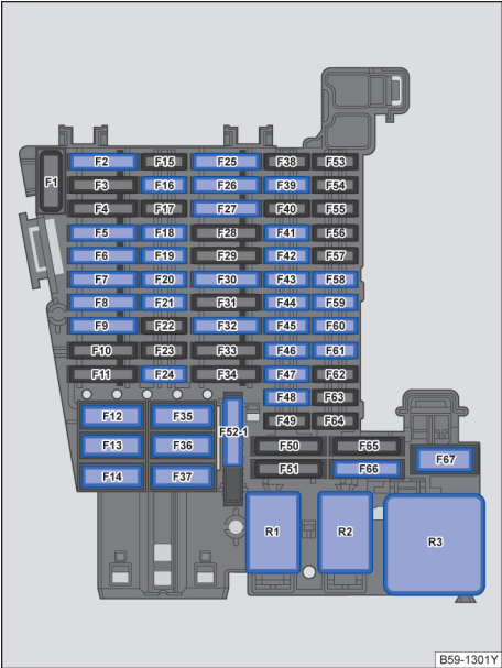
图 207 仪表板中：保险丝分配
