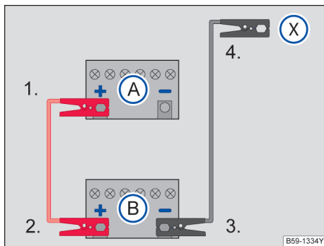
图 210 跨接电缆连接示意图
