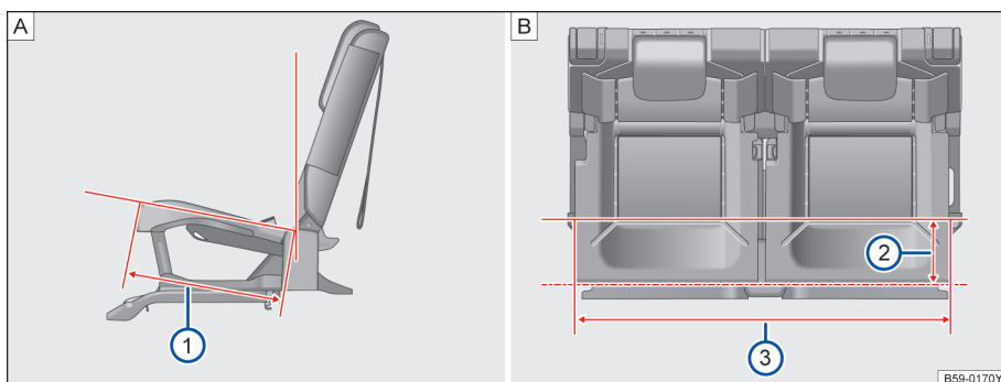
图 100 第三排座椅座宽和坐垫深
