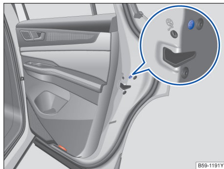
图 58 右侧后车门端面处的应急上锁装置（由橡胶密封件遮盖着）
