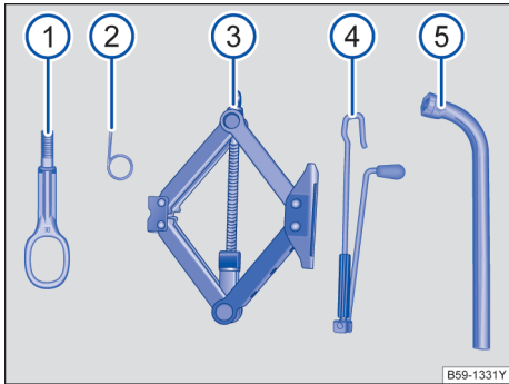
图 202 随车工具的组件
