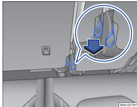
图 83 第二排座椅：第三排座椅紧急登出功能的锁止拉扣。
