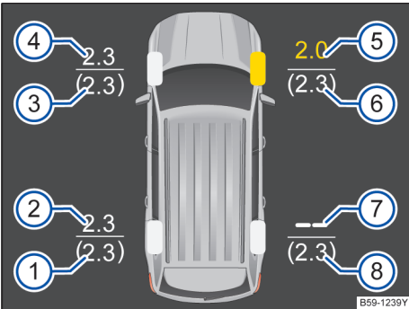
图 223 组合仪表中显示屏上：当前轮胎压力
