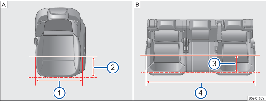
图 105 前排及第二排座椅座宽
