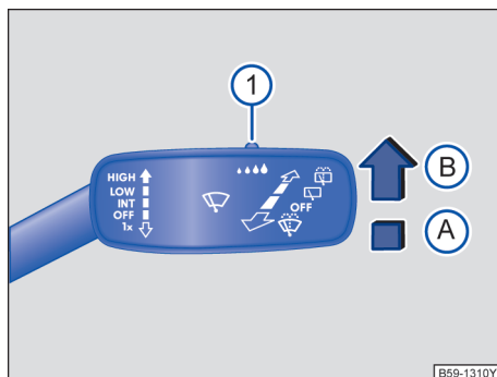
图 117 车窗玻璃刮水器操作杆：调节雨量传感器
