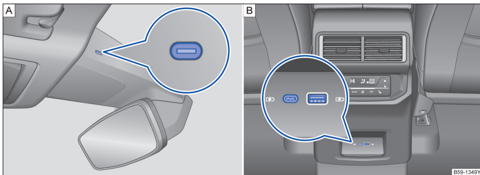
图 177 [A]. 车顶 Type-C 插口（视装备而定） [B]. 中控台后部分的 USB、Type-C 插口
