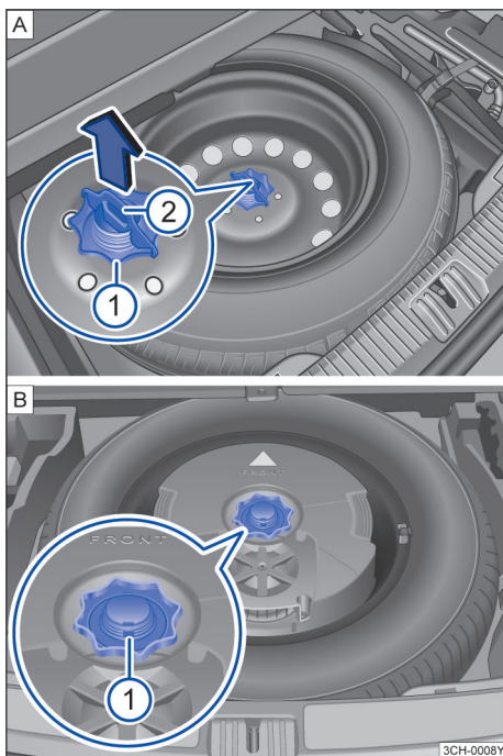
图 226 行李厢内：备用轮胎固定手轮（类型 A 和类型 B）
