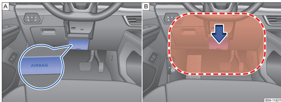
图 41 驾驶员侧：膝部安全气囊安装位置及作用范围
