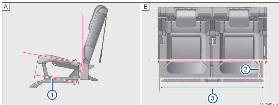
图 106 第三排座椅座宽和坐垫深
