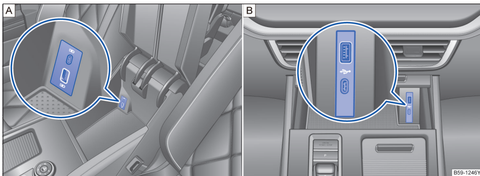
图 176 [A]. 前部中央扶手储物盒内的 USB、Type-C 插口 [B]. 前部储物盒内的 USB、Type-C 插口
