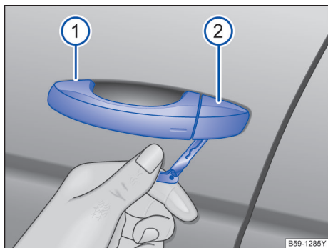
图 57 取下在驾驶员车门内车门锁的盖罩
