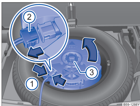
图 235 行李厢内：拆下重低音扬声器
