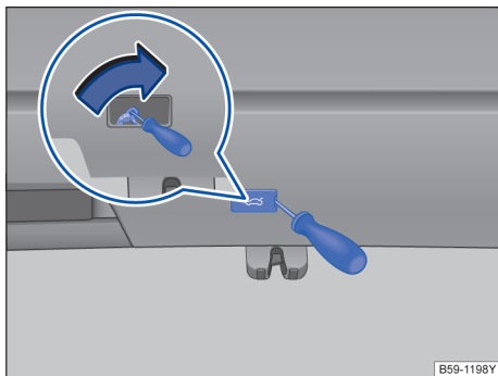
图 68 在行李厢中：行李厢盖的应急解锁机构
